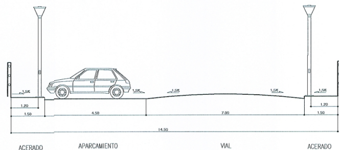
SECCION E-E'
