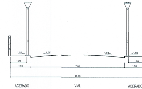
SECCION G-G'
