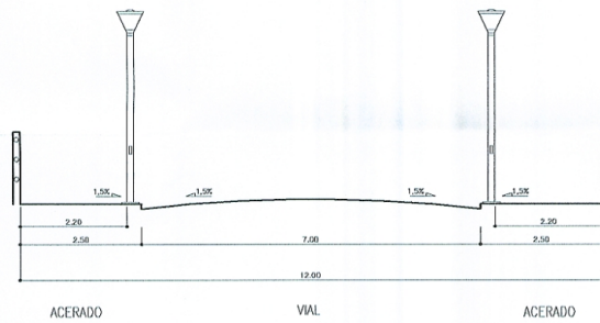
SECCION B-B'
