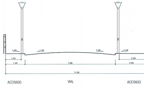
SECCION F-F'
