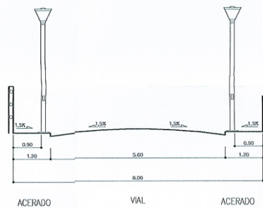
SECCION A-A'
