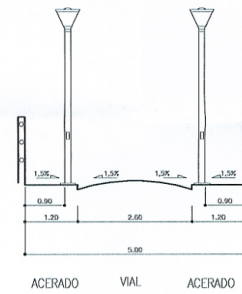
SECCION C-C'
