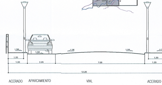
SECCION D-D'
